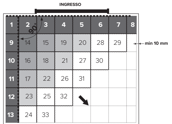
Fig. n. 2 Posa Fortelock INVISIBLE, INVISIBLE XL, BUSINESS
