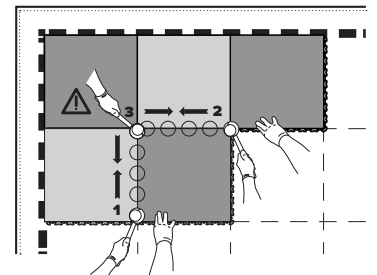
Fig. n. 4 Metodo di posa delle piastrelle INVISIBLE, INVISIBLE XL, BUSINESS
