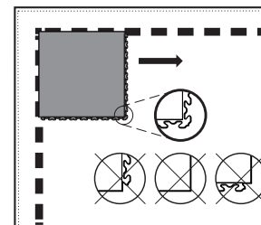
Fig. n. 3 Direzione di posa delle piastrelle INVISIBLE, INVISIBLE XL, BUSINESS
